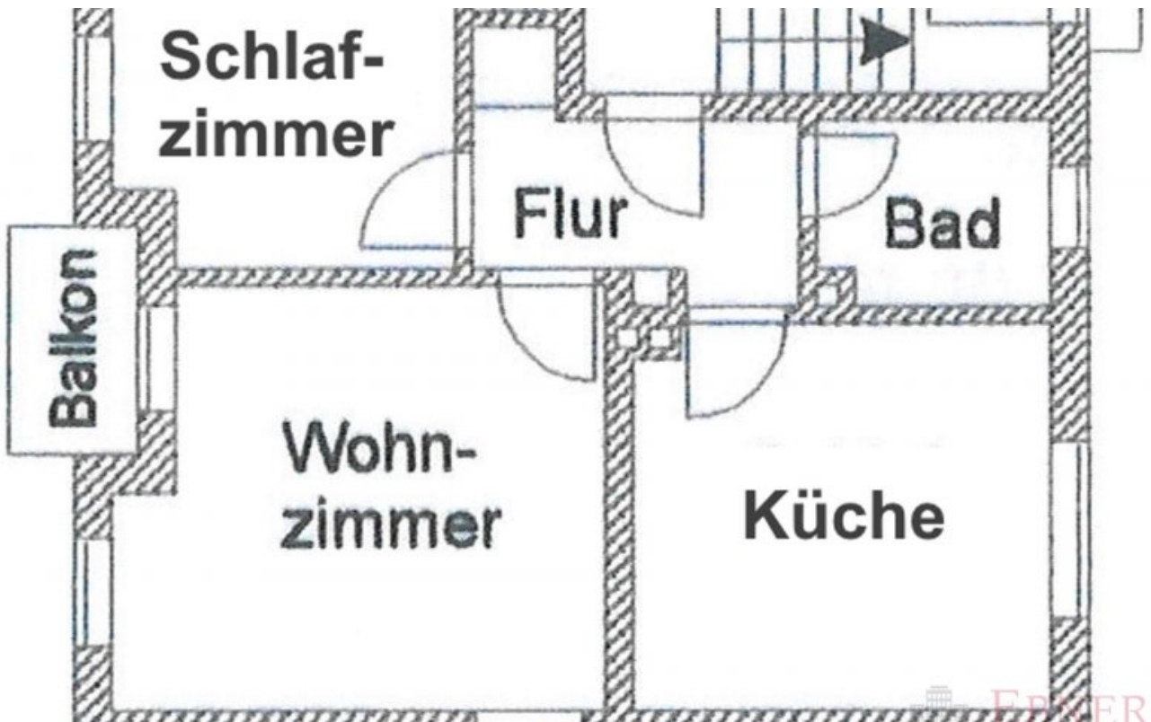
1336 Grundriss (Grundriss)
